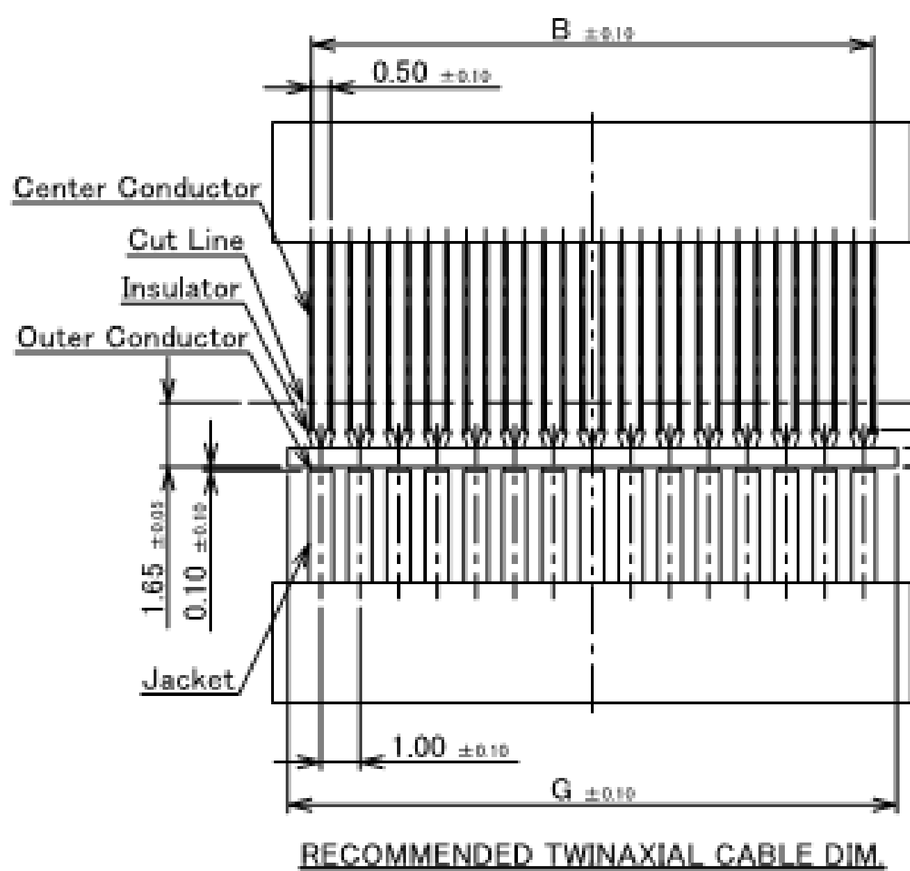
TWINAXIAL CABLE AWG #40
