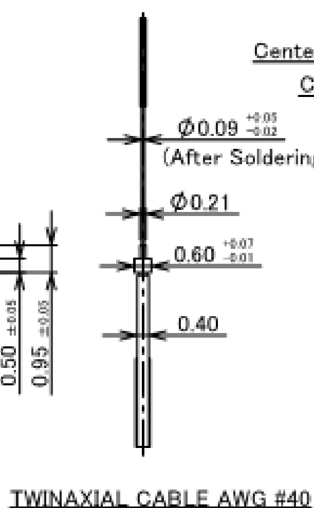
TWINAXIAL CABLE AWG #40
